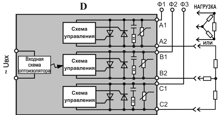
D – реле Ф1, Ф2, Ф3 - фазы коммутируемого напряжения
