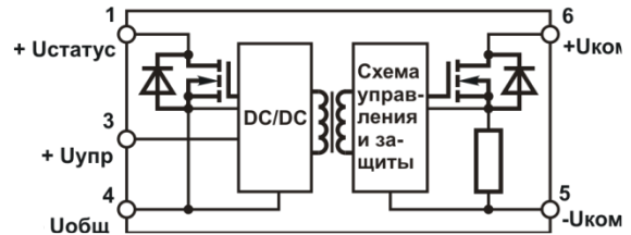
Электрическая схема
