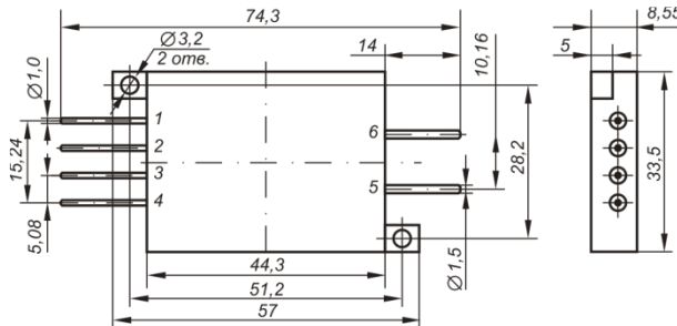
Габаритный чертеж корпуса
