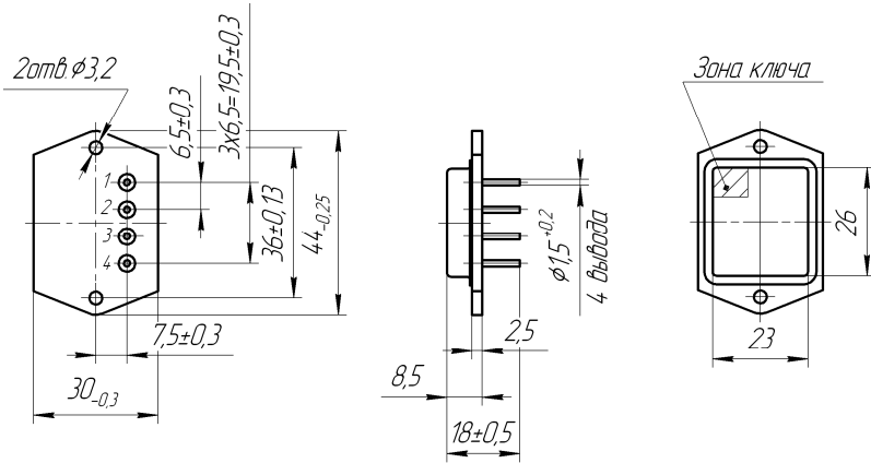
Габаритный чертеж
